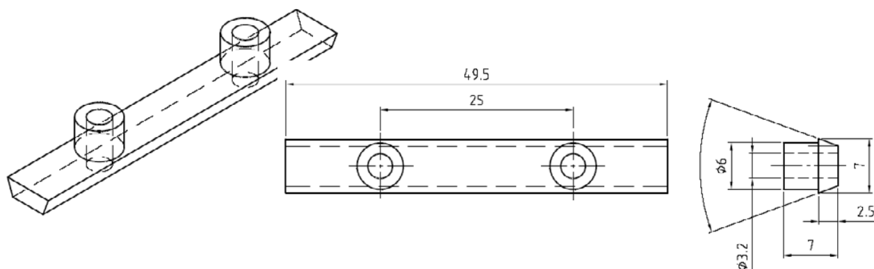
EINLEGESCHIENE AT10 AUS POLYAMID ODER MESSING MIT M4 L=50MM
